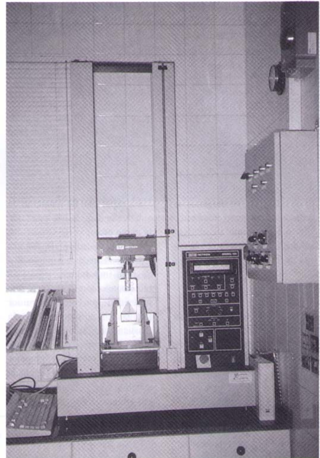
Aparato para determinar la dureza de la carne.
